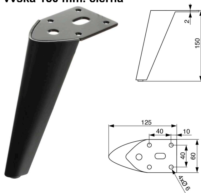
Nábytková nožička kovová SL049, výška 150 mm, čierna
