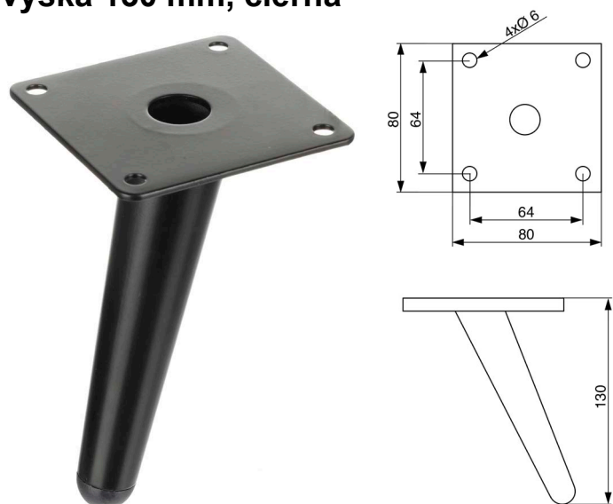
Nábytková nožička kovová SL052, výška 130 mm, čierna
