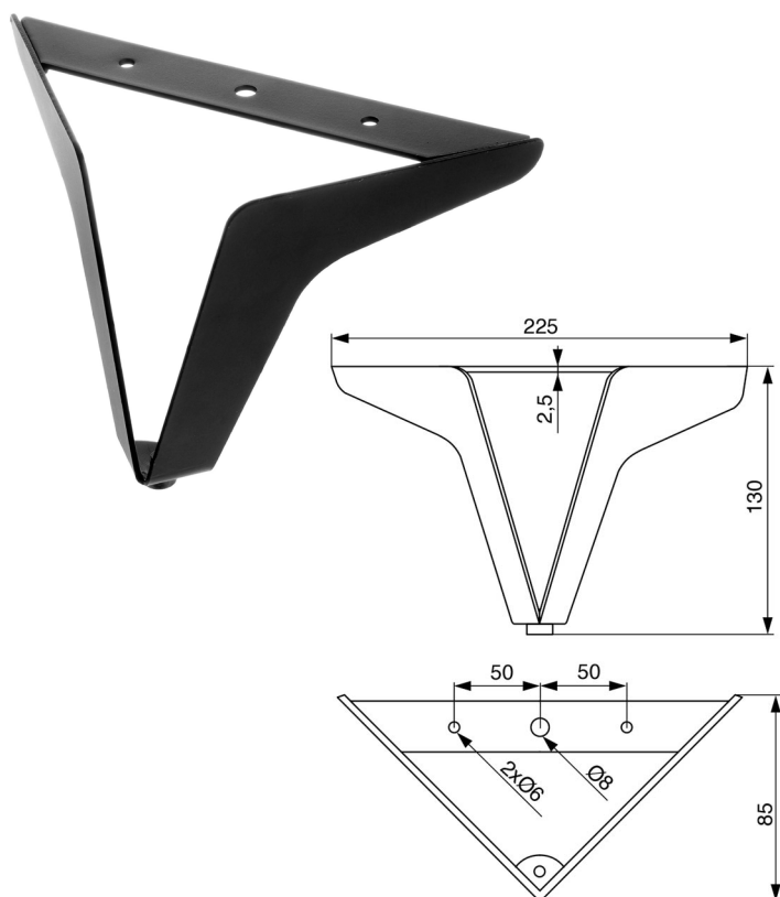
Nábytková nožička kovová SL047, výška 130 mm, čierna
